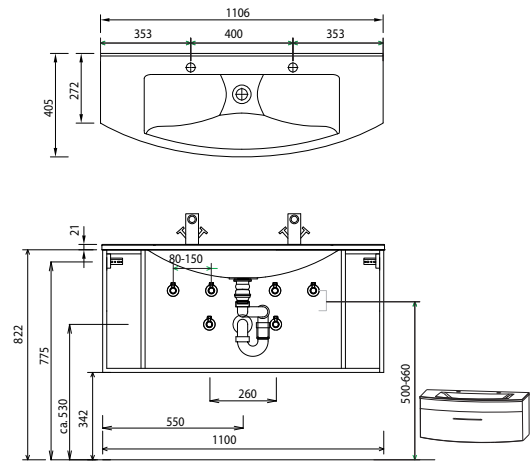
WMC R41D S1 für WUA 3511 7
