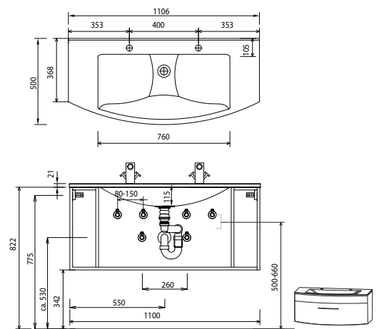
WMC R51D S1 für WUA 3511 T7
