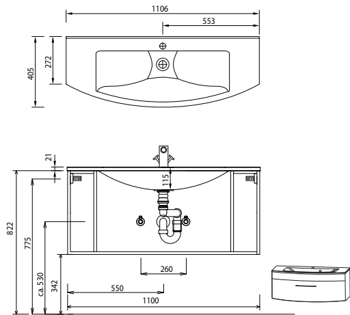
WMC R411 1 für WUA 3511 7
