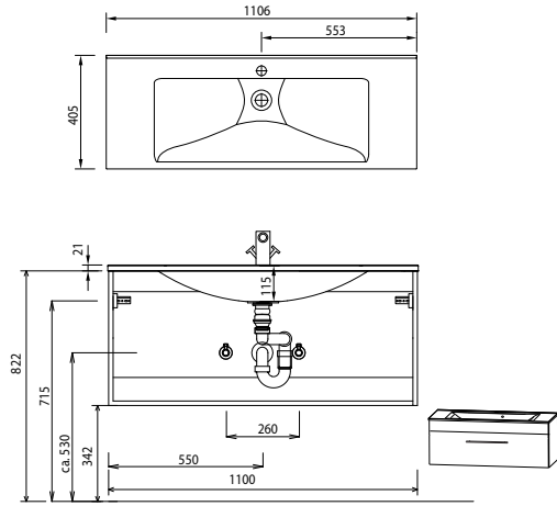
WMC G411 1 für WUA 3811 7
